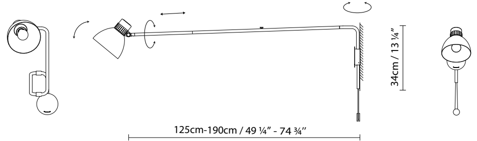
W125
